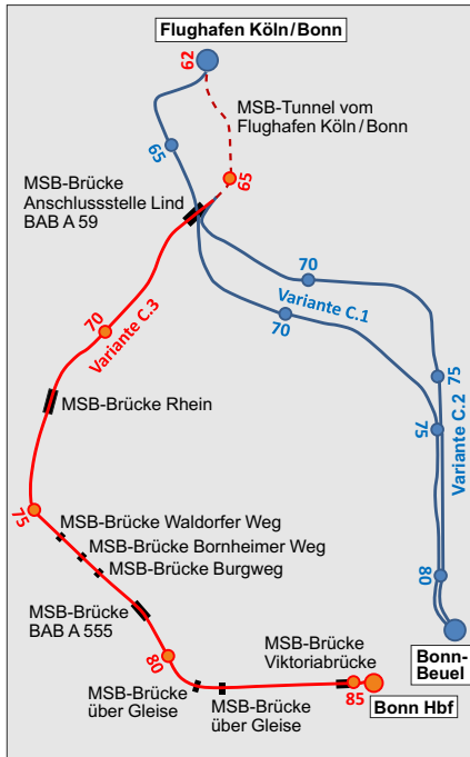
Übersichtslageplan Trassenvarianten Flughafen Köln/Bonn - Bonn Hbf
