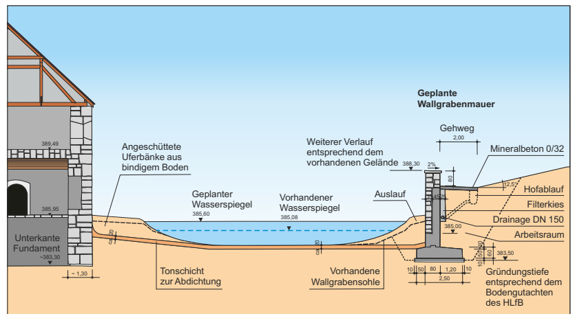
Schnitt durch die neue Wallmauer
