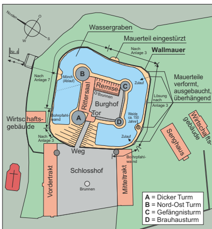
Grundriss der Burganlage
