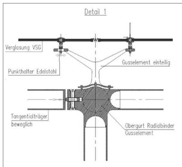
Detail 1 Dachinnenrand mit Verglasung
